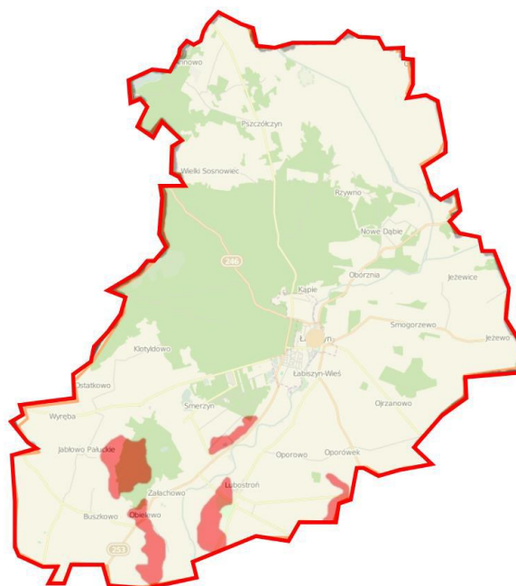
Ryc. 37. Obszary predysponowane do występowania ruchów masowych na terenie gminy Łabiszyn.
