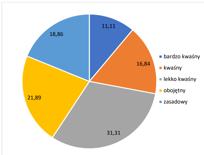
Ryc. 32. Odczyn pH zbadanych gleb z terenu gminy Łabiszyn (udział %)
