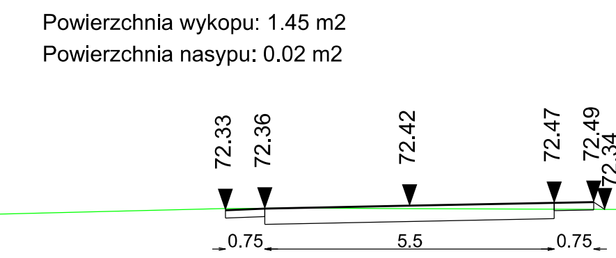
Przekroje poprzeczne 1+000.00
