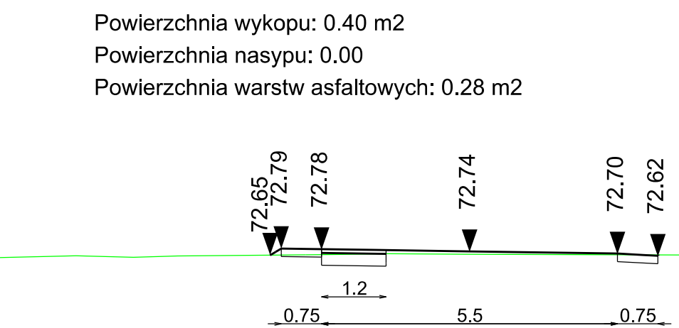
Przekroje poprzeczne 1+375.64
