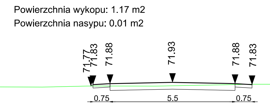
Przekroje poprzeczne 0+650.00
