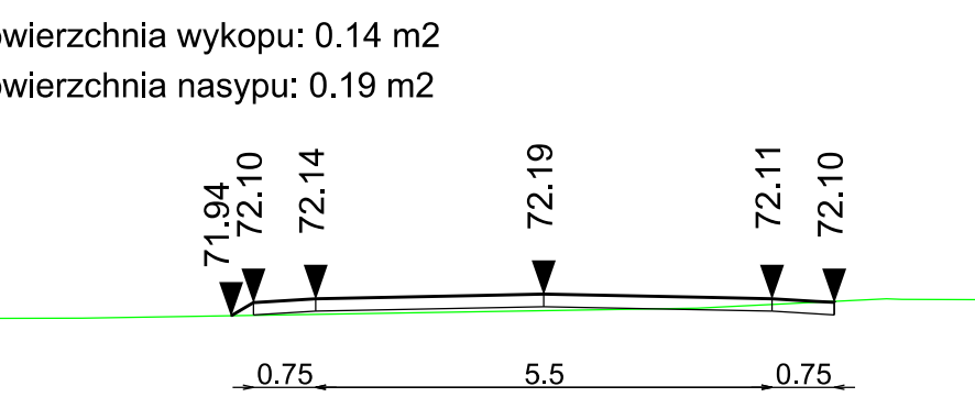
zestroje porzeczne 0+900.00
