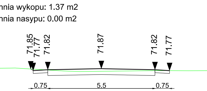
rzekroje poprzeczne 0+750.00
