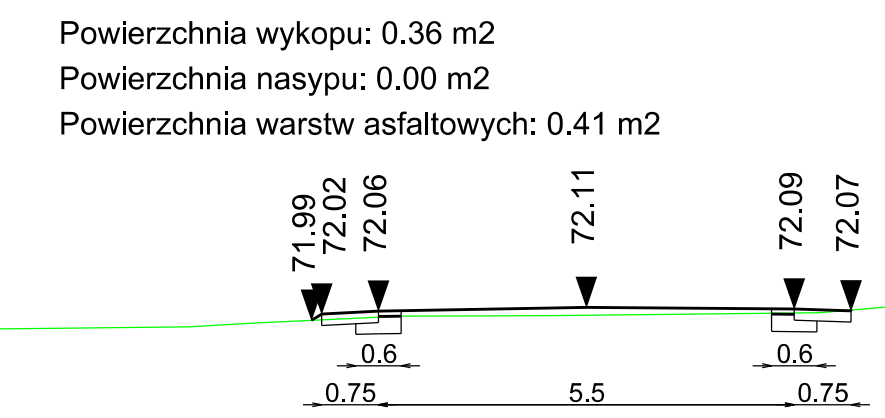
Przekroje poprzeczne 1+250.00
