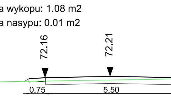
Przekroje poprzeczne 0+893.73
