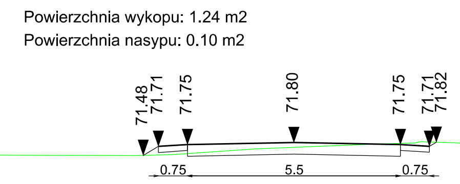
Przekroje poprzeczne 0+700.00
