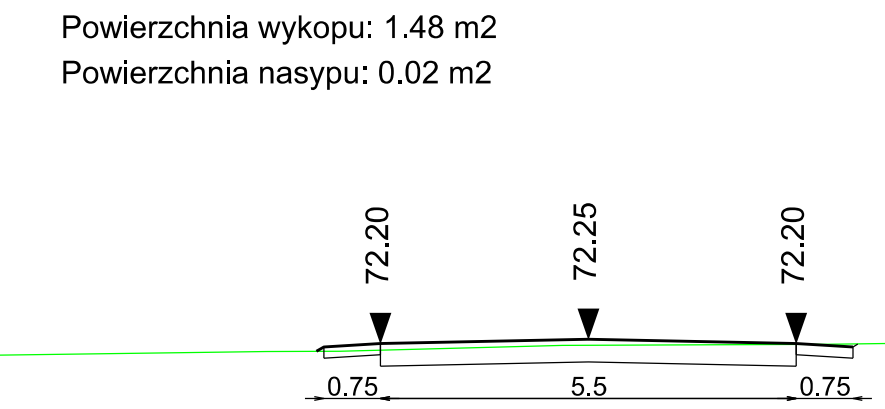
Przekroje poprzeczne 0+941.00
