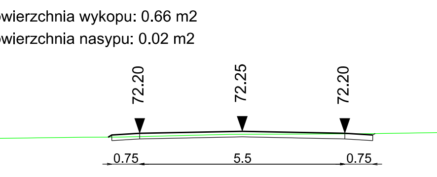
zestawienie przekrojów poprzecznych 0+941.00
