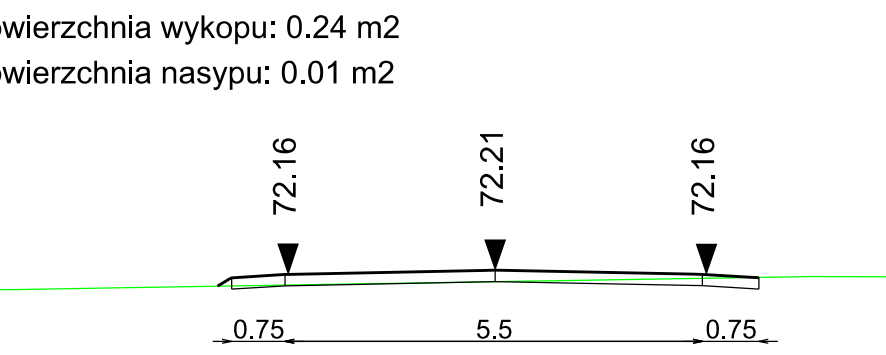
zestroje porzeczne 0+893.73
