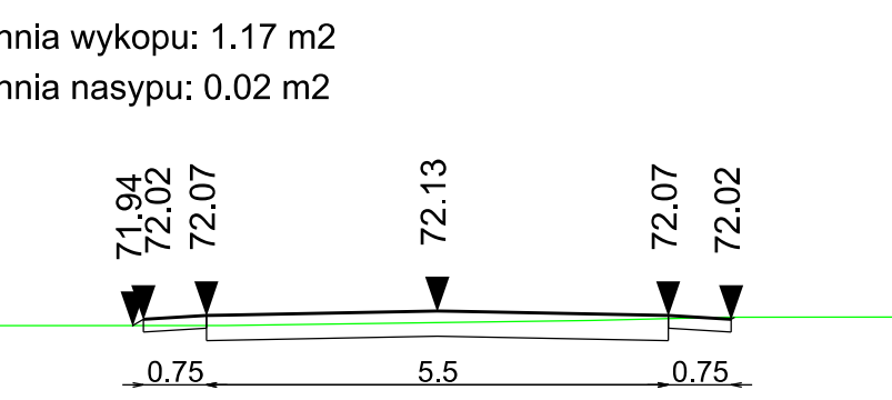
rzekroje poprzeczne 0+850.00
