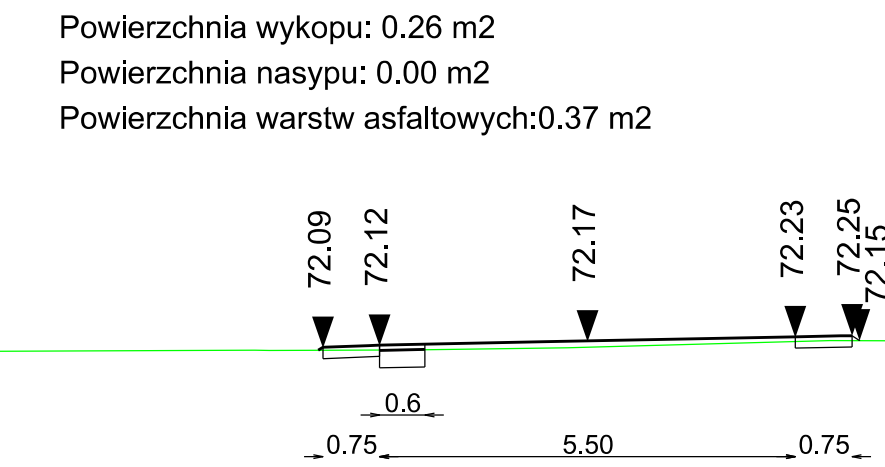
Przekroje poprzeczne 1+200.00
