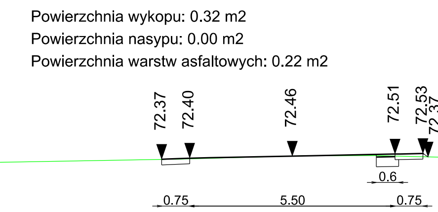
Przekroje poprzeczne 1+100.00
