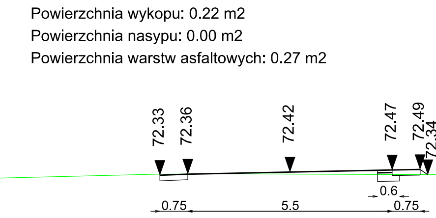
Przekroje poprzeczne 1+050.00
