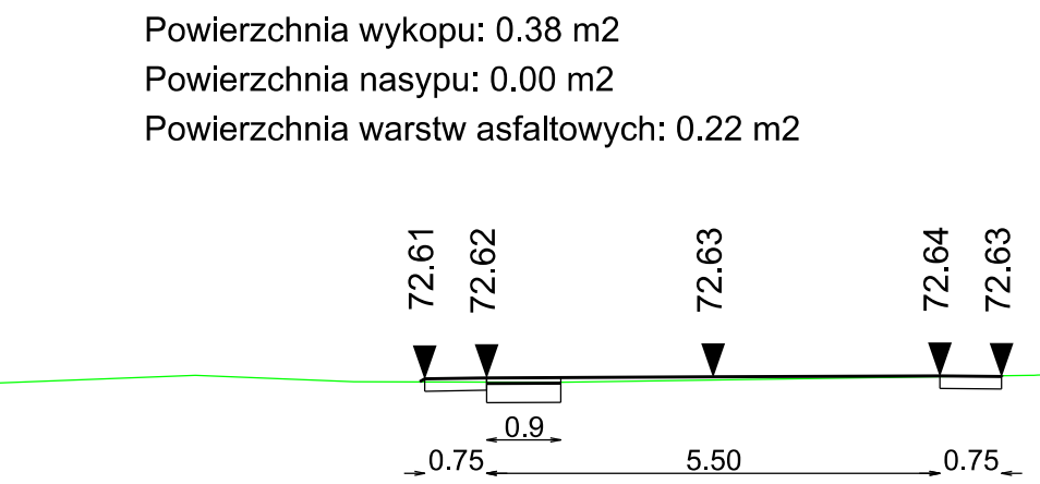
Przekroje poprzeczne 1+350.00
