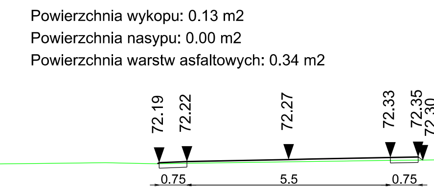
Przekroje poprzeczne 1+050.00
