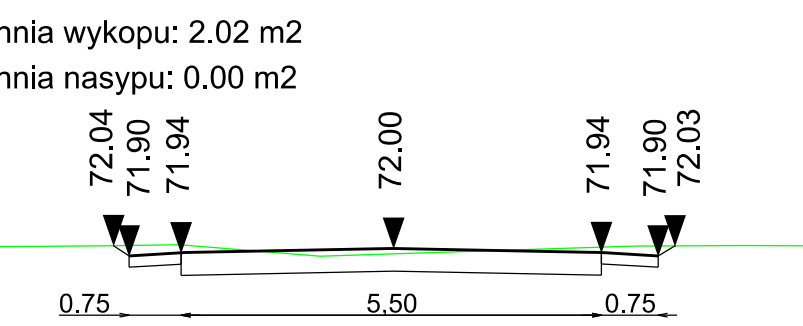
rzekroje porzeczne 0+800.00
