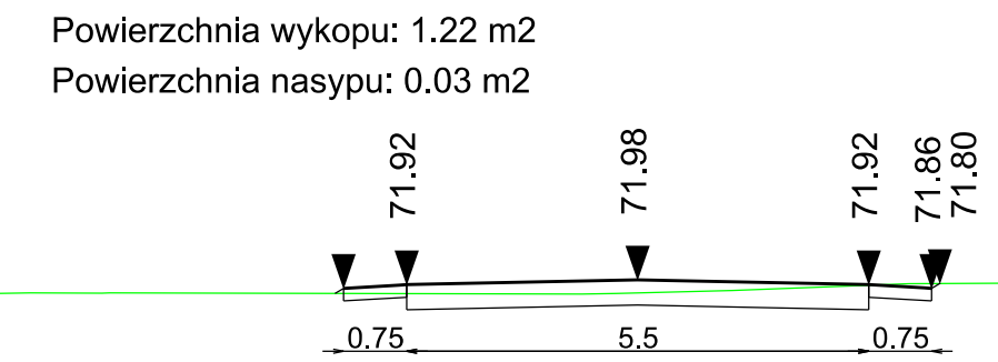
Przekroje poprzeczne 0+630.00
