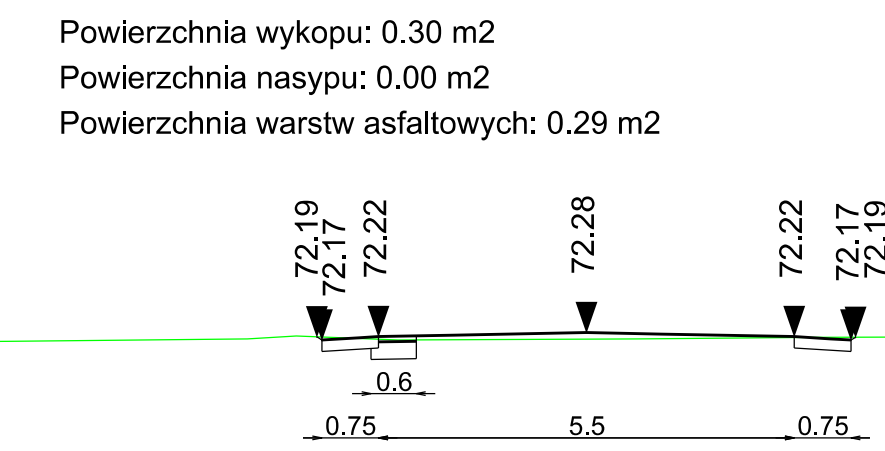
Przekroje poprzeczne 1+250.00
