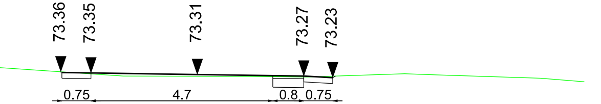
Przekroje poprzeczne 0+250.00
