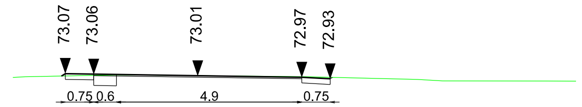
Przekroje poprzeczne 0+050.00
