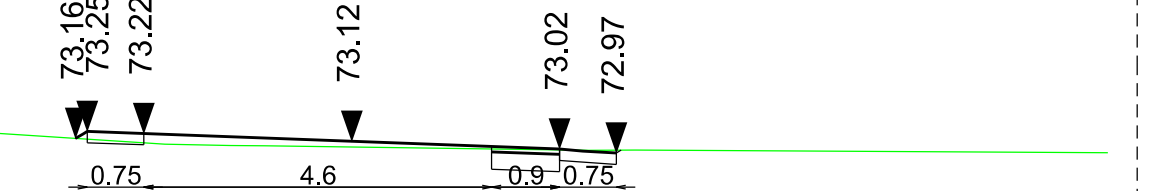
Przekroje poprzeczne 0+314.00
