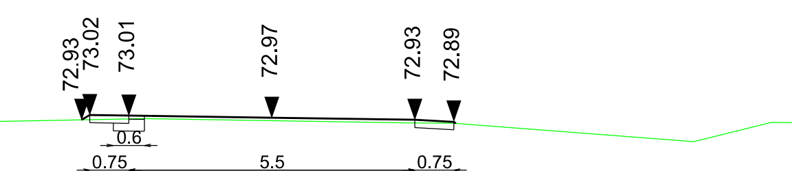
Przekroje poprzeczne 0+100.00
