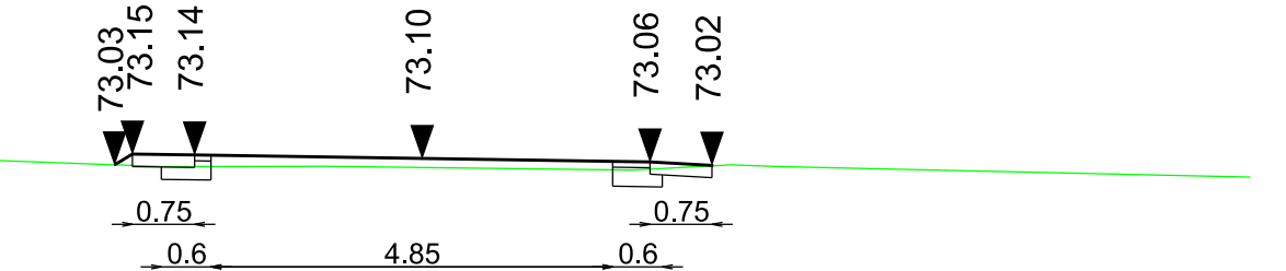
Przekroje poprzeczne 0+200.00
