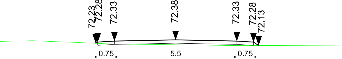
Przekroje poprzeczne 0+560.00
