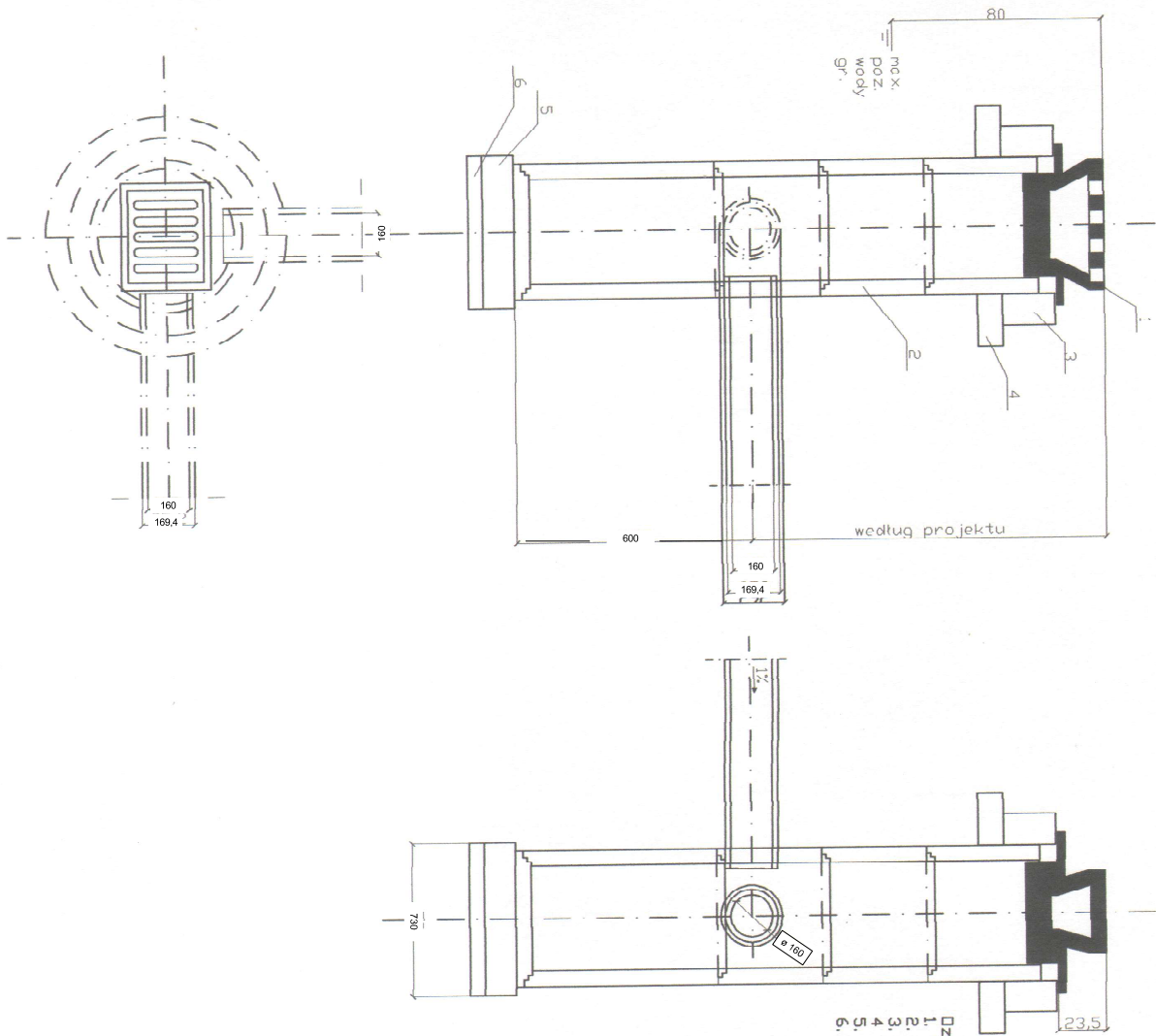
Studzienka ściekowa Ø500mm z osadnikiem
