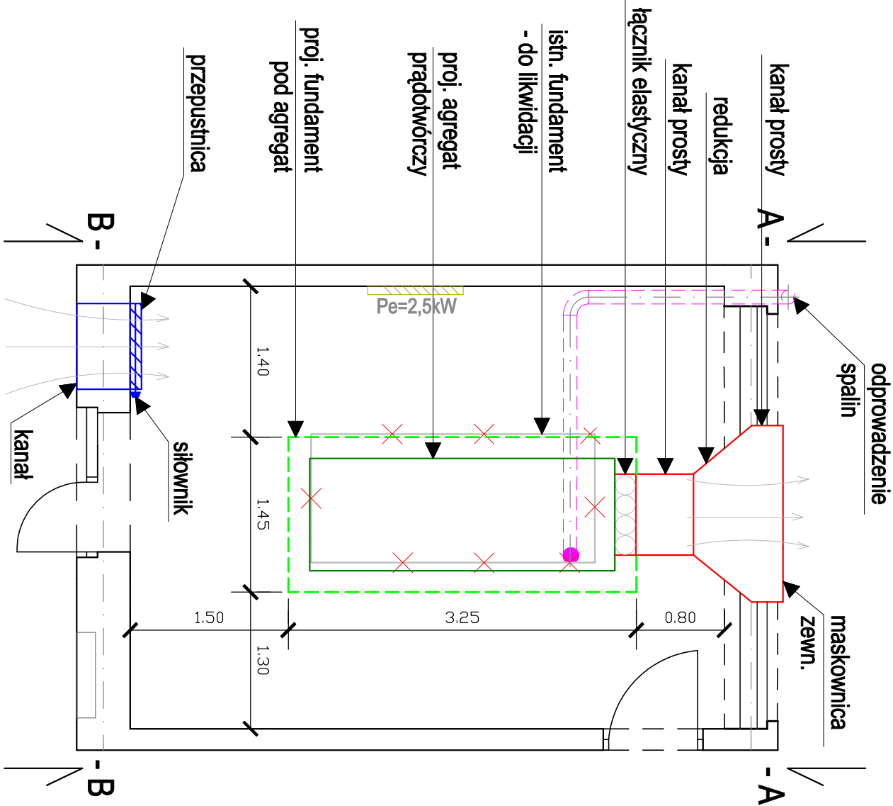
RZUT
