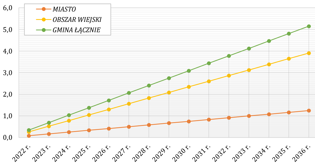
Wykres 26. Prognozowany przyrost zapotrzebowania na moc ciepłą (c.o.) w sektorze mieszkalnictwa na terenie Gminy Łabiszyn związany z oddawaniem do użytkowania nowych budynków mieszkalnych w perspektywie do 2036 r. [MW]
