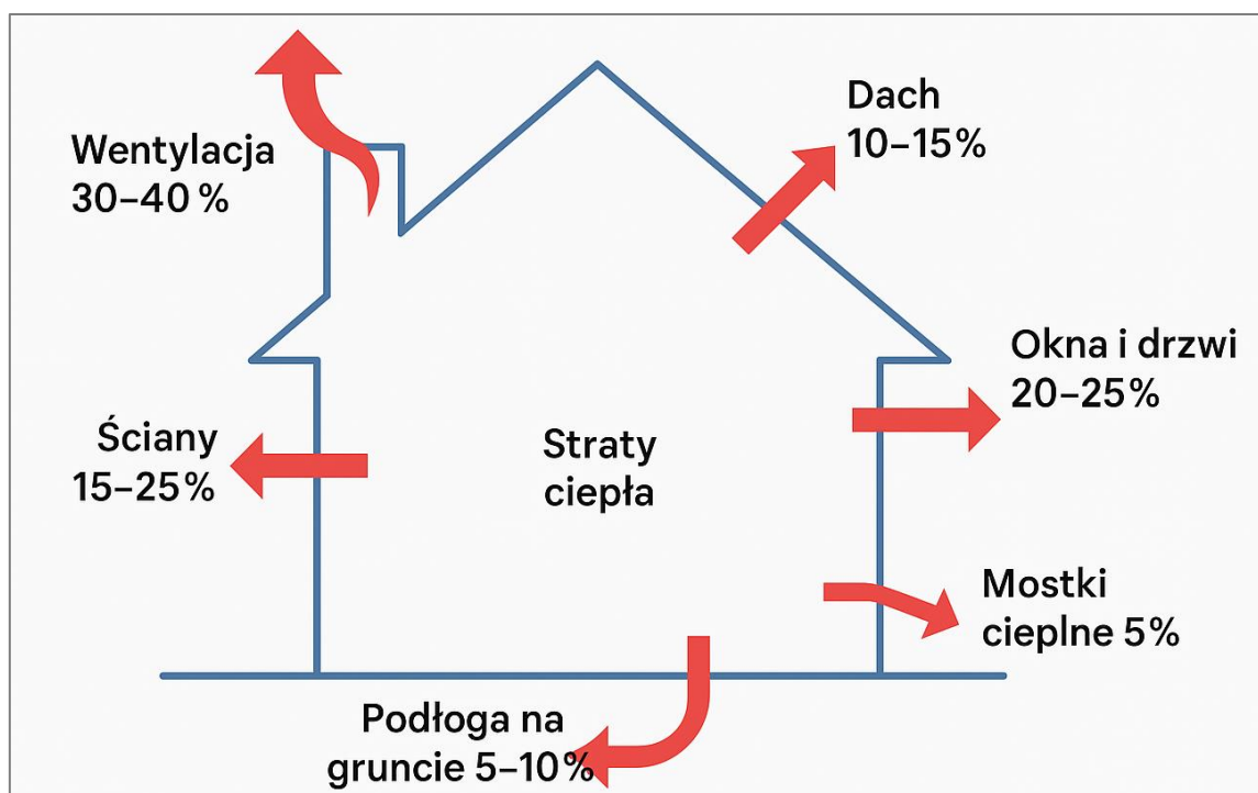
Rysunek 6. Rozkład poszczególnych strat ciepła przez przenikanie przez przegrody i wentylację w bilansie energetycznym budynku mieszkalnego jednorodzinnego Źródło: opracowanie własne
