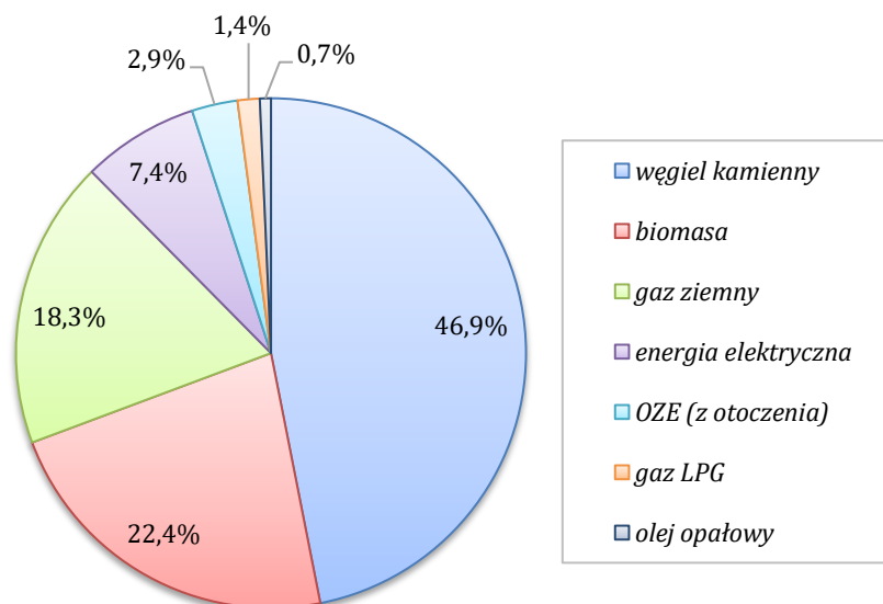
Wykres 17. Udział poszczególnych nośników energii w zużyciu ciepła (pokryciu potrzeb grzewczych) w sektorze mieszkalnictwa na terenie gminy Łabiszyn
