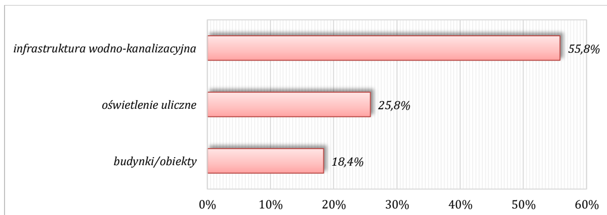
Wykres 36. Struktura zużycia energii elektrycznej w sektorze komunalnym na terenie gminy Łąbiszyn
