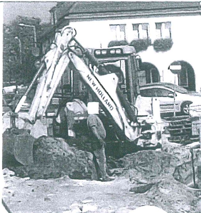
6, 7 – pracownicy (fot. 6) i (fot. 7) nie stosowali podczas pracy na budowie spodni roboczych posiadających właściwości ochronne oraz kamizelki ochronnej; nie stosował obuwia roboczego
