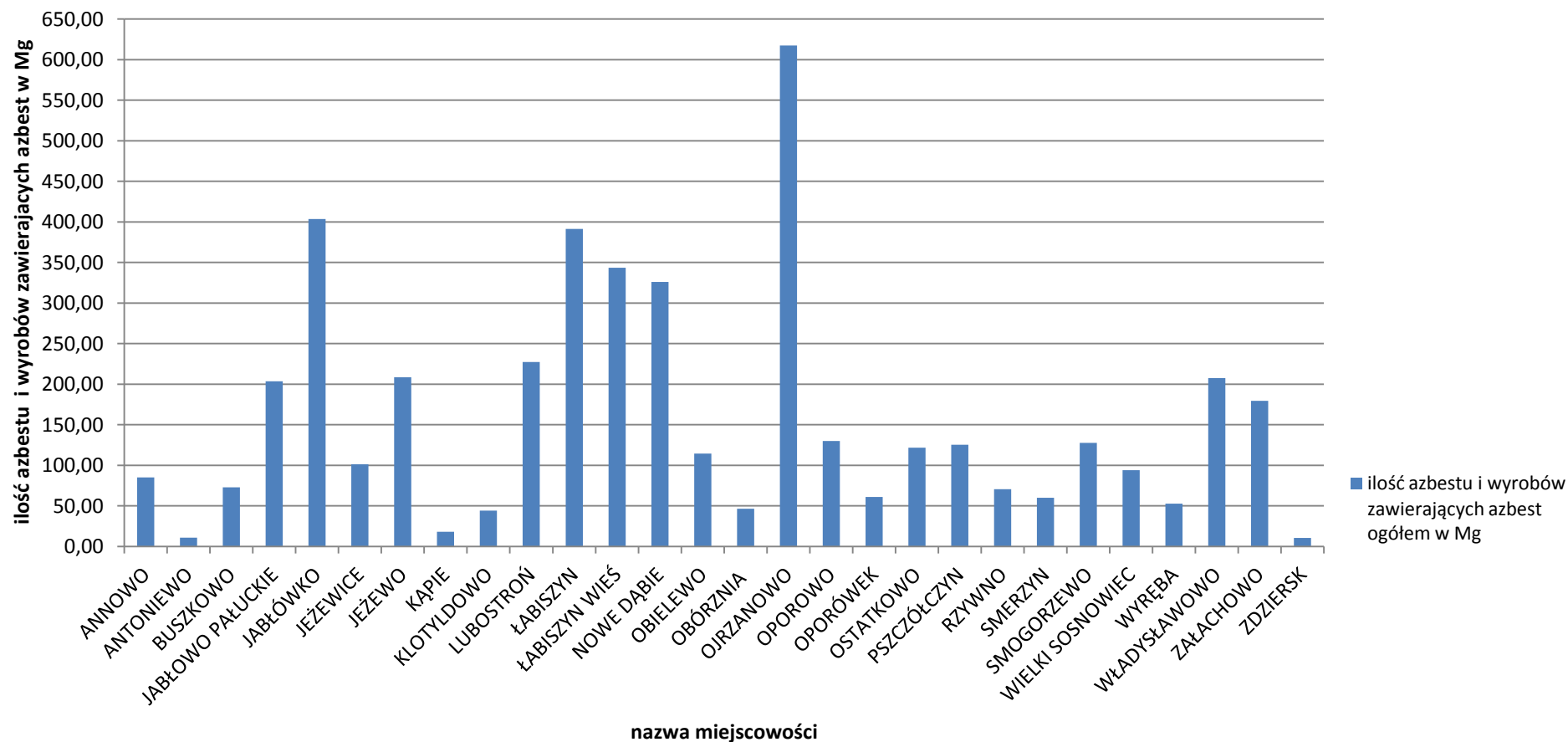
Wykres2. Ilość zinwentaryzowanego azbestu i wyrobów zawierających azbest ogółem w poszczególnych miejscowościach Gminy Łabiszyn
